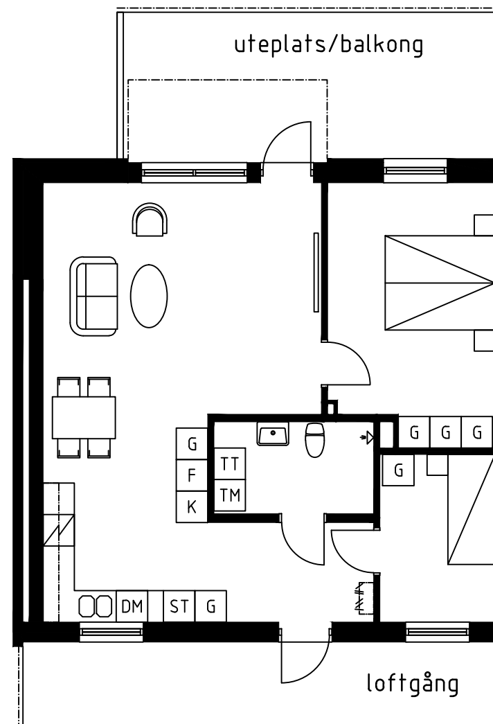
Planlösning 3 ROK
